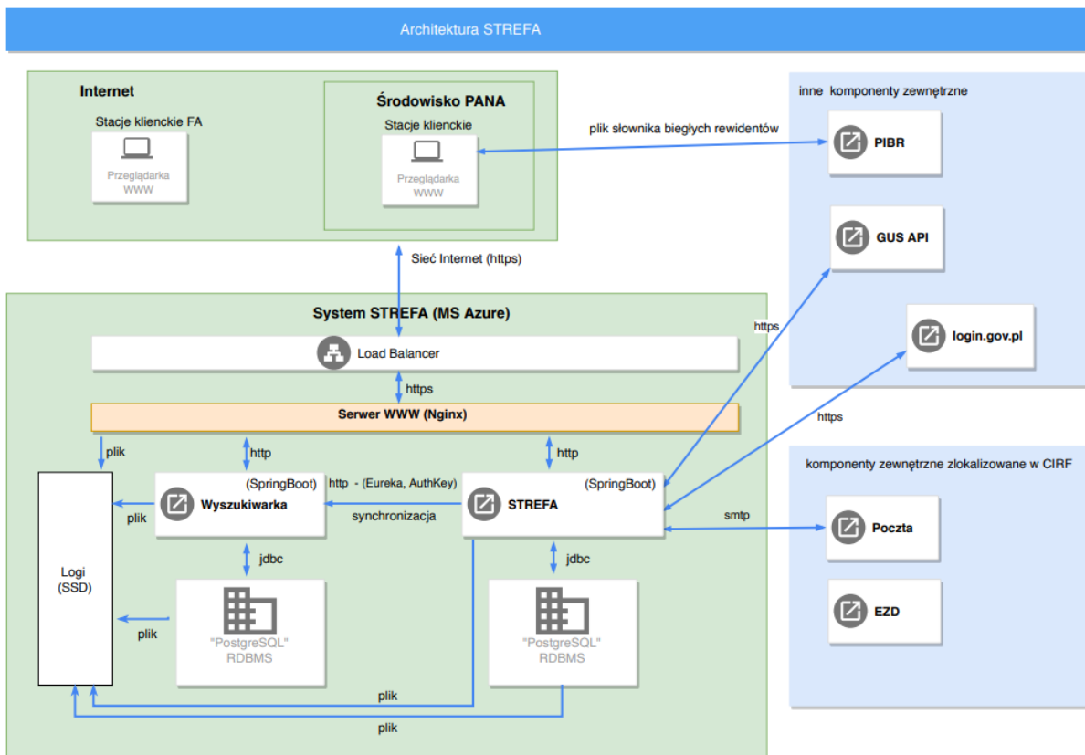
Rysunek 2 Diagram prezentujący architekturę Systemu STREFA
