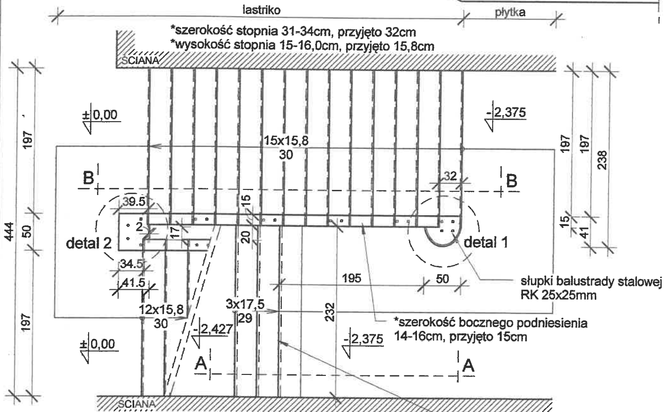
RZUT KLATKI SCHOD. piwnica - parter *szerokość stopnia 29-30cm, przyjęto 29cm *wysokość stopnia 17,5-18cm, przyjęto 17,5cm stopnie w piwnicy zakończone kątownikiem stalowym dł. 200cm
