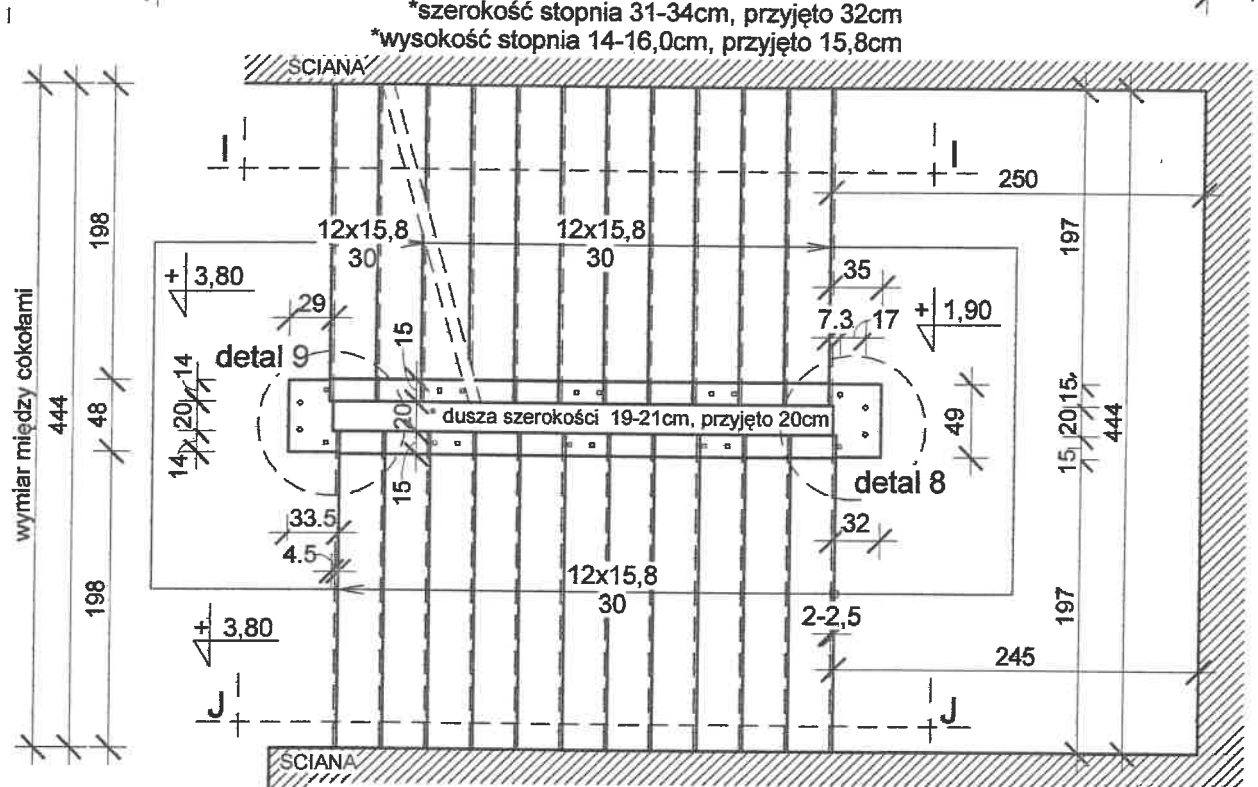
RZUT KLATKI SCHOD. parter - I piętro
