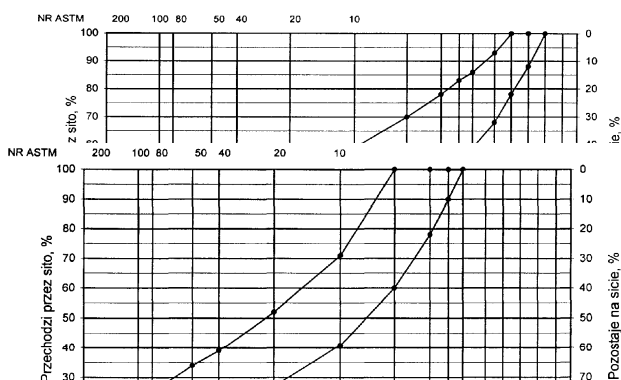
Rys. 1 Krzywe graniczne uziarnienia mieszanki mineralnej BA od 0 do 8mm, od 0 do 6,3 mm do warstwy ścieralnej nawierzchni drogi o obciążeniu ruchem KR1 lub KR2
