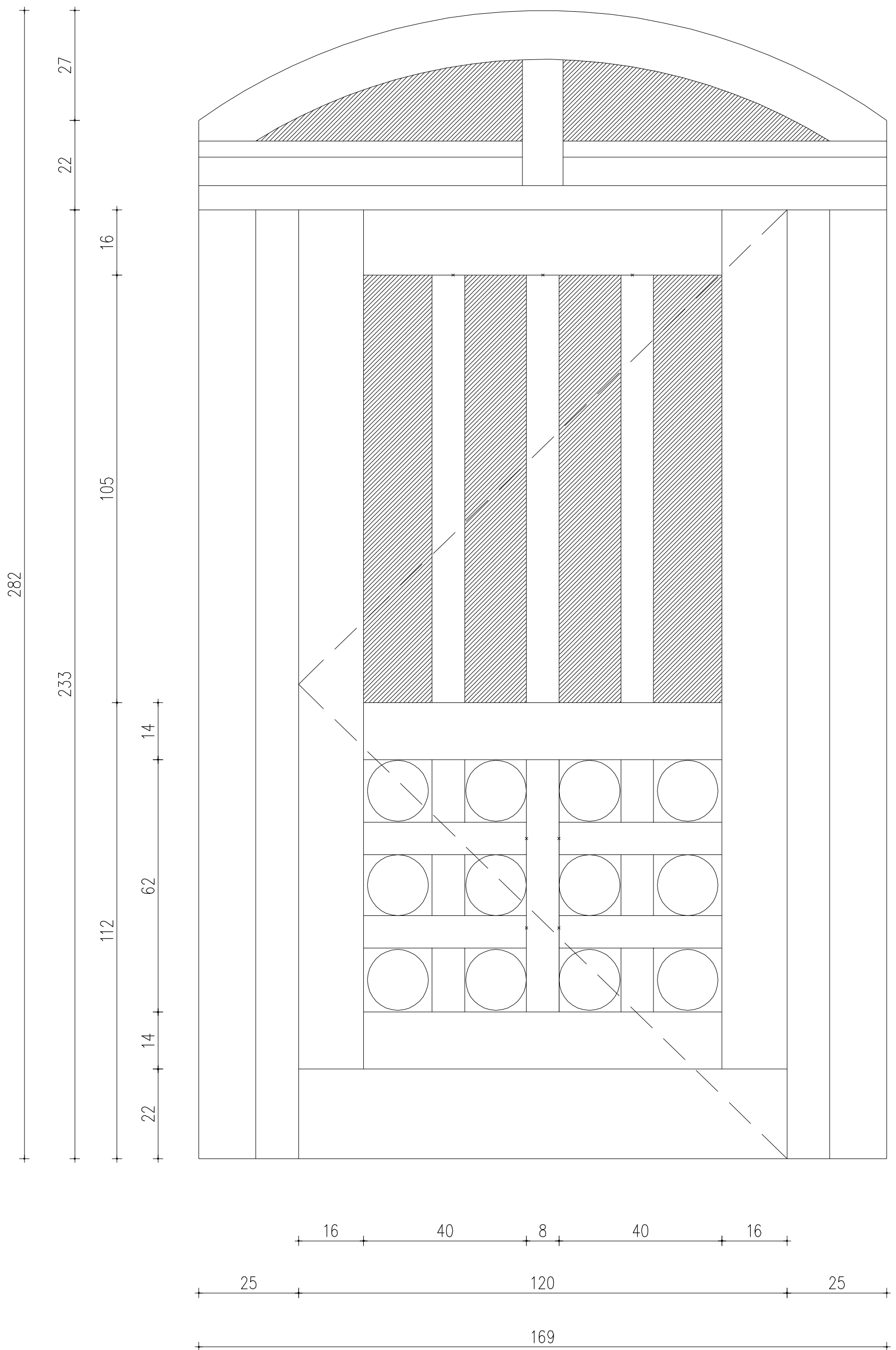
GŁÓWNE DRZWI WYJŚCIOWE NA OGRÓD SKRZYDŁO 120/233 cm DETAL ANALOGISZNIE DO ISTNIEJĄCYCH
