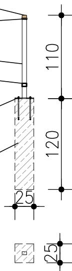
WIDOK FUNDAMENTU - GORA
