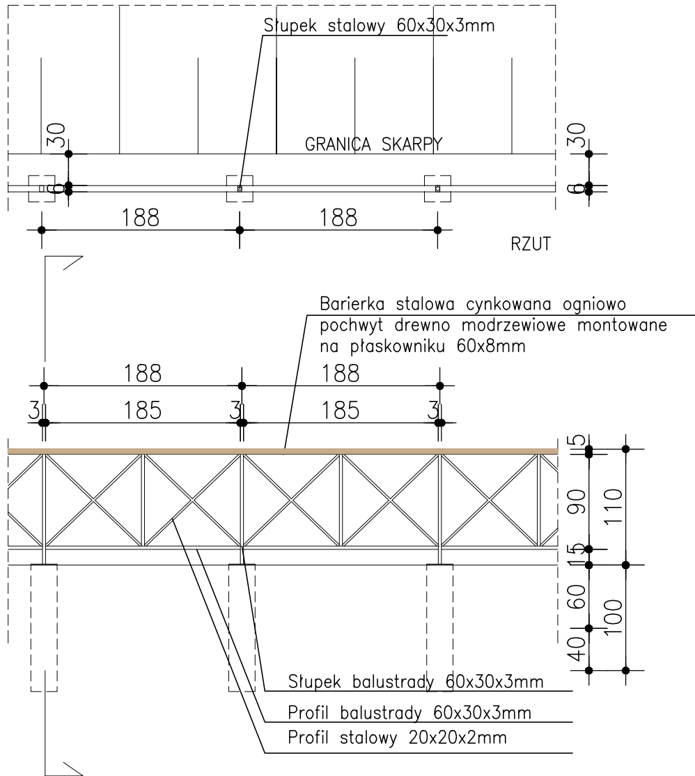
WIDOK - FRONT
