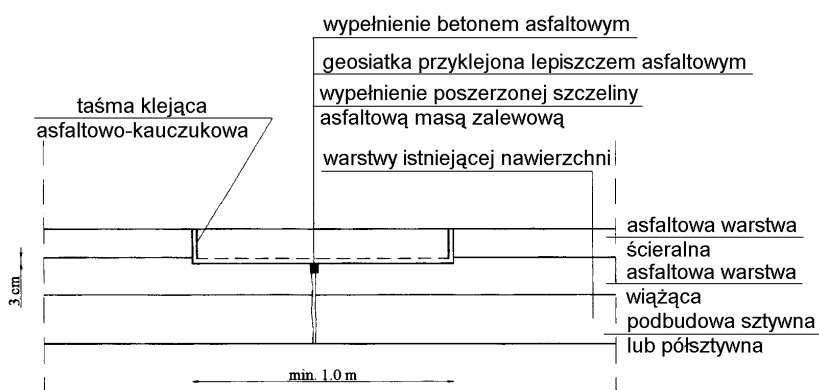
Rys. 1. Naprawa płytko pojedynczego pęknięcia odbitego, gdy krawędzie pęknięcia są dobrze podparte - w istniejącej warstwie ścieralnej
