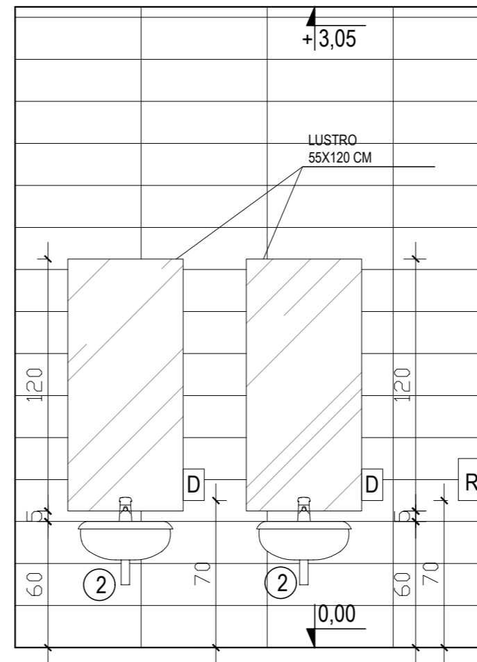
WIDOK D
