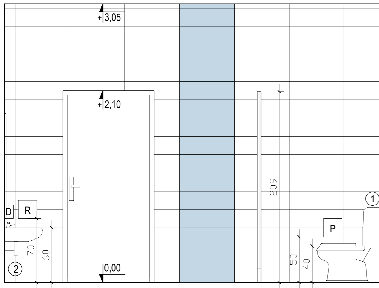
WIDOK C
