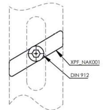
schemat łączenia śrub scheme of tightening screws
