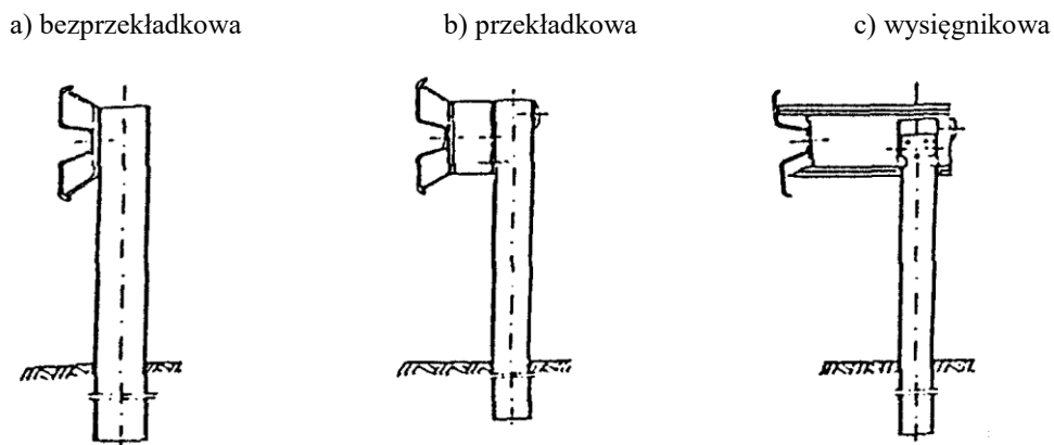
Załącznik 11.3. Zasady określania wysokości prowadnicy bariery nad poziomem terenu, Wg [32]
