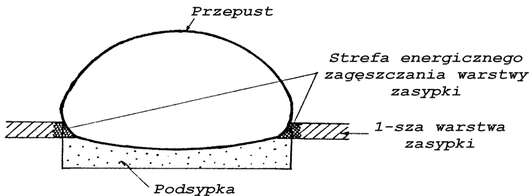
Rys. nr 2. Zagęszczenie zасыпки w strefach pachwinowych.
