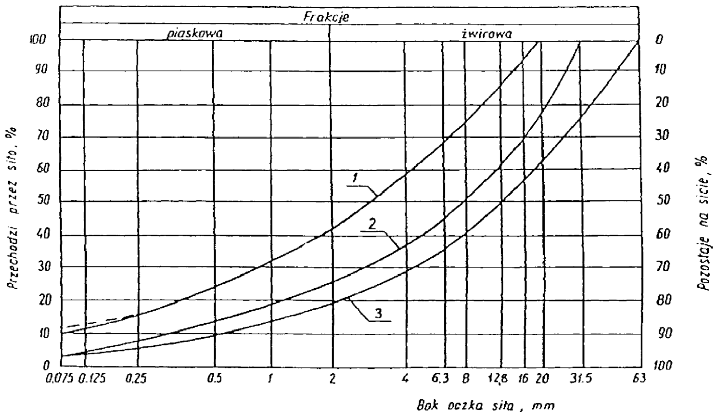
Rysunek 1. Pole dobrego uziarnienia kruszyw przeznaczonych na podbudowy wykonywane metodą stabilizacji mechanicznej 1-3 kruszywo na podbudowę pomocniczą (dolną warstwę) 0-31,5 mm
