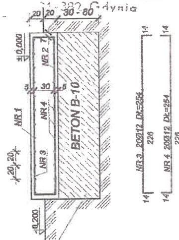
PRZEKRÓJ B-B
