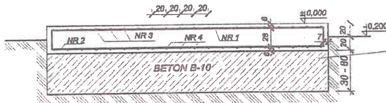
PRZEKRÓJ A-A
