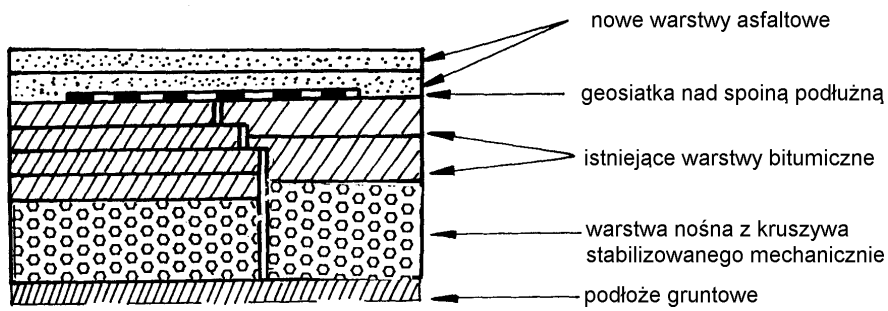
Rys. 1. Wzmocnienie nawierzchni asfaltowej w strefie poszerzenia nawierzchni
