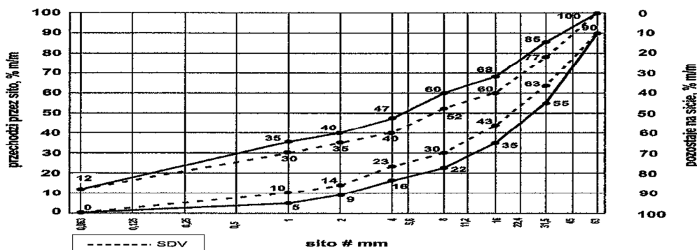
Rys. 1. Krzywe graniczne uziarnienia mieszanki kruszywa niezwiązanego 0/63 mm do warstw podbudowy pomocniczej
