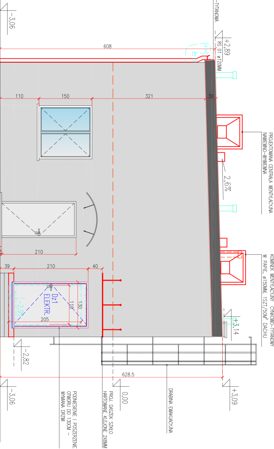
ELEWACJA ZACHODNIA
