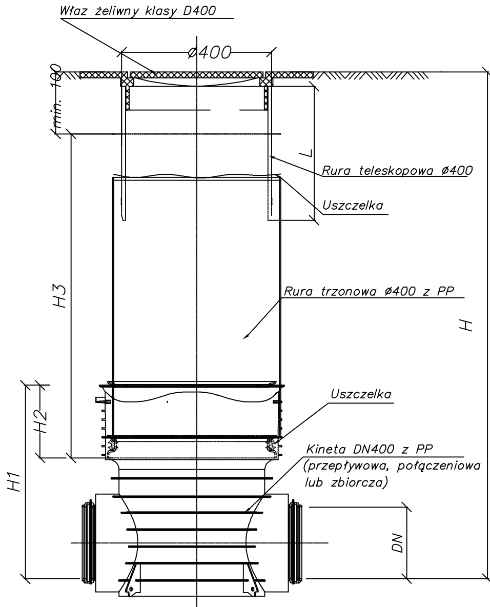
Studzienka rewizyjna DN400 z rurą teleskopową i włazem żeliwnym typu ciężkiego klasy D400
