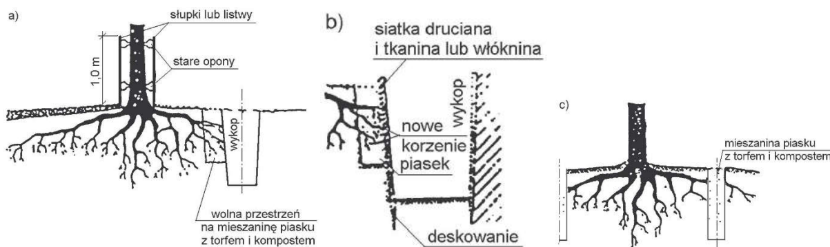
Rys. 1. Wykonywanie wykopów instalacyjnych w obrębie strefy korzeniowej drzew
