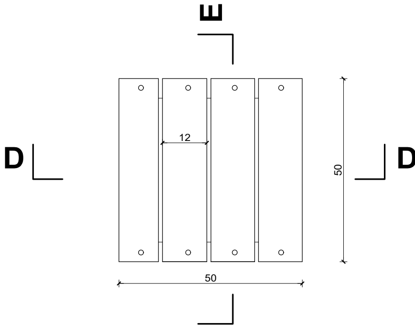
Siedzisko - widok z góry, skala 1:10
