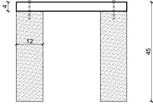
Siedzisko - przekrój E-E, skala 1:10
