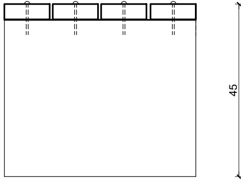
Siedzisko - przekrój D-D, skala 1:10
