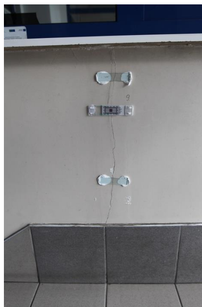
Pomieszczenie 2 – parter, zarysowanie ścian
