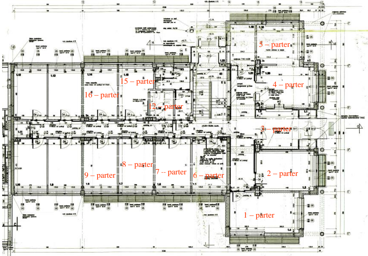
Rzut parteru budynku Komisariatu Policji
