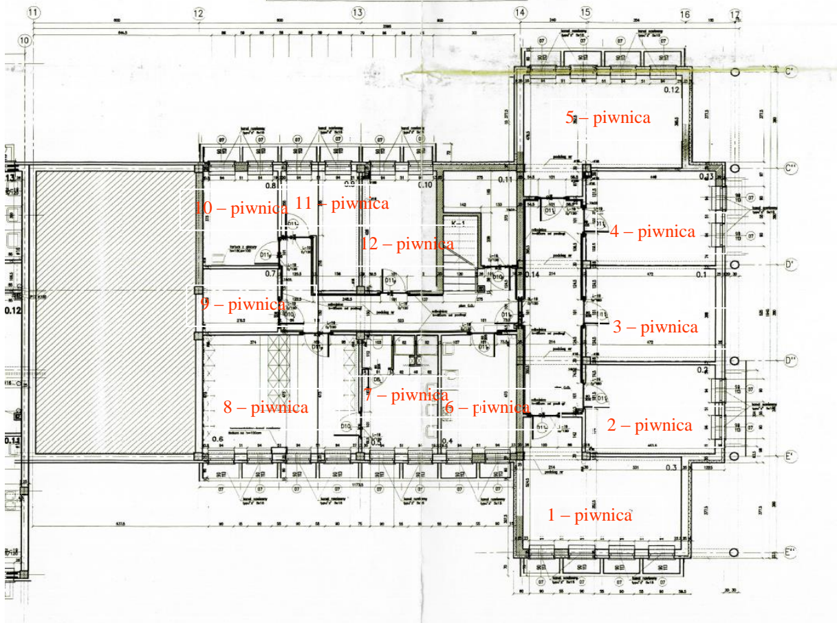
Rzut piwnic budynku Komisariatu Policji
