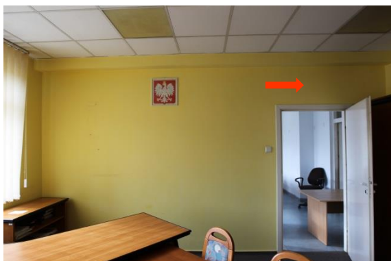
Pomieszczenie 2 – I piętro, zarysowania ściany nad drzwiami wew. między pomieszczeniami 1 i 2
