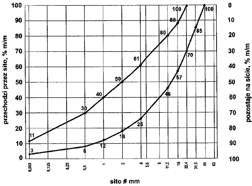
Rys. 1 Krzywe graniczne uziarnienia mieszanki mineralnej 0/31,5
