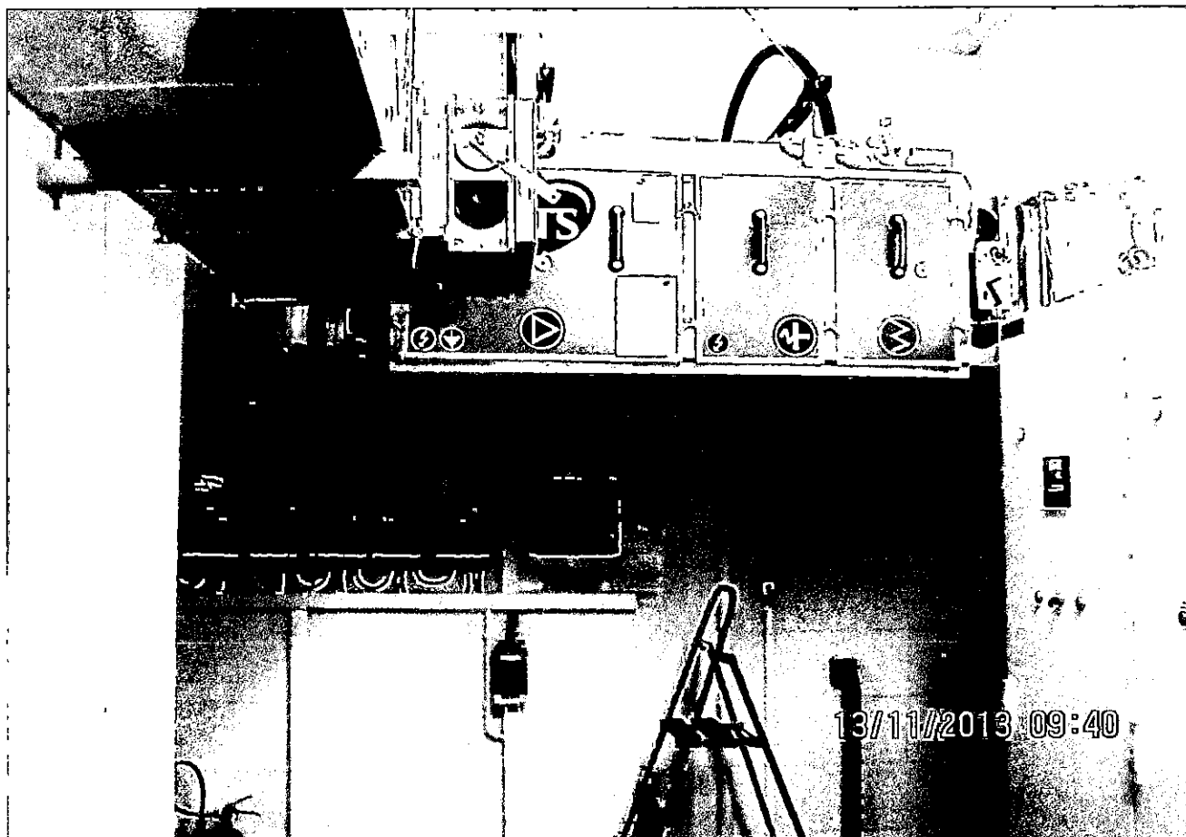
FOT.2 WIDOK CENTRALI NAWIEWNEJ NR 2
