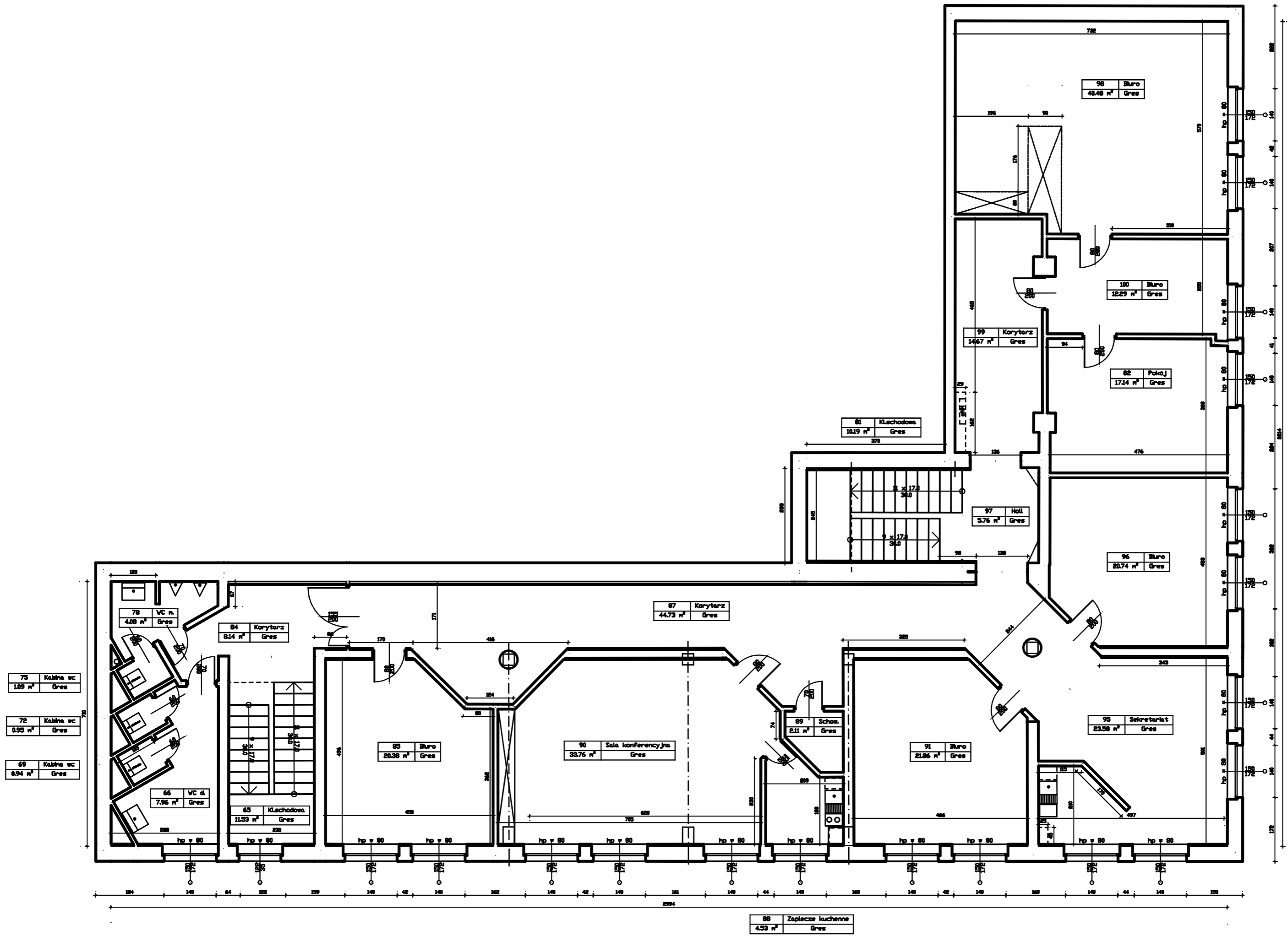
RZUT II PIĘTRA
