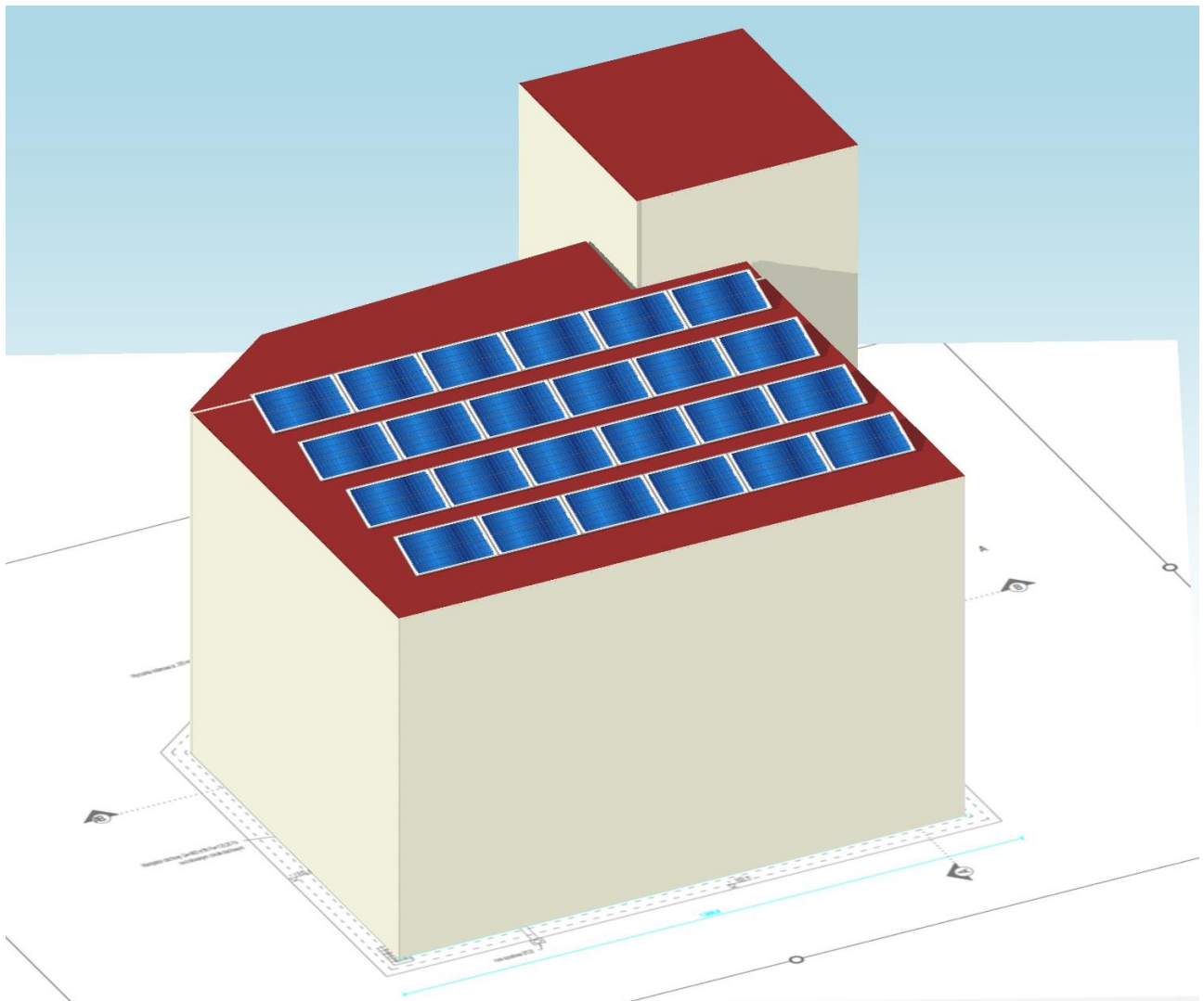
Rysunek 3: Realistyczny widok instalacji systemu
