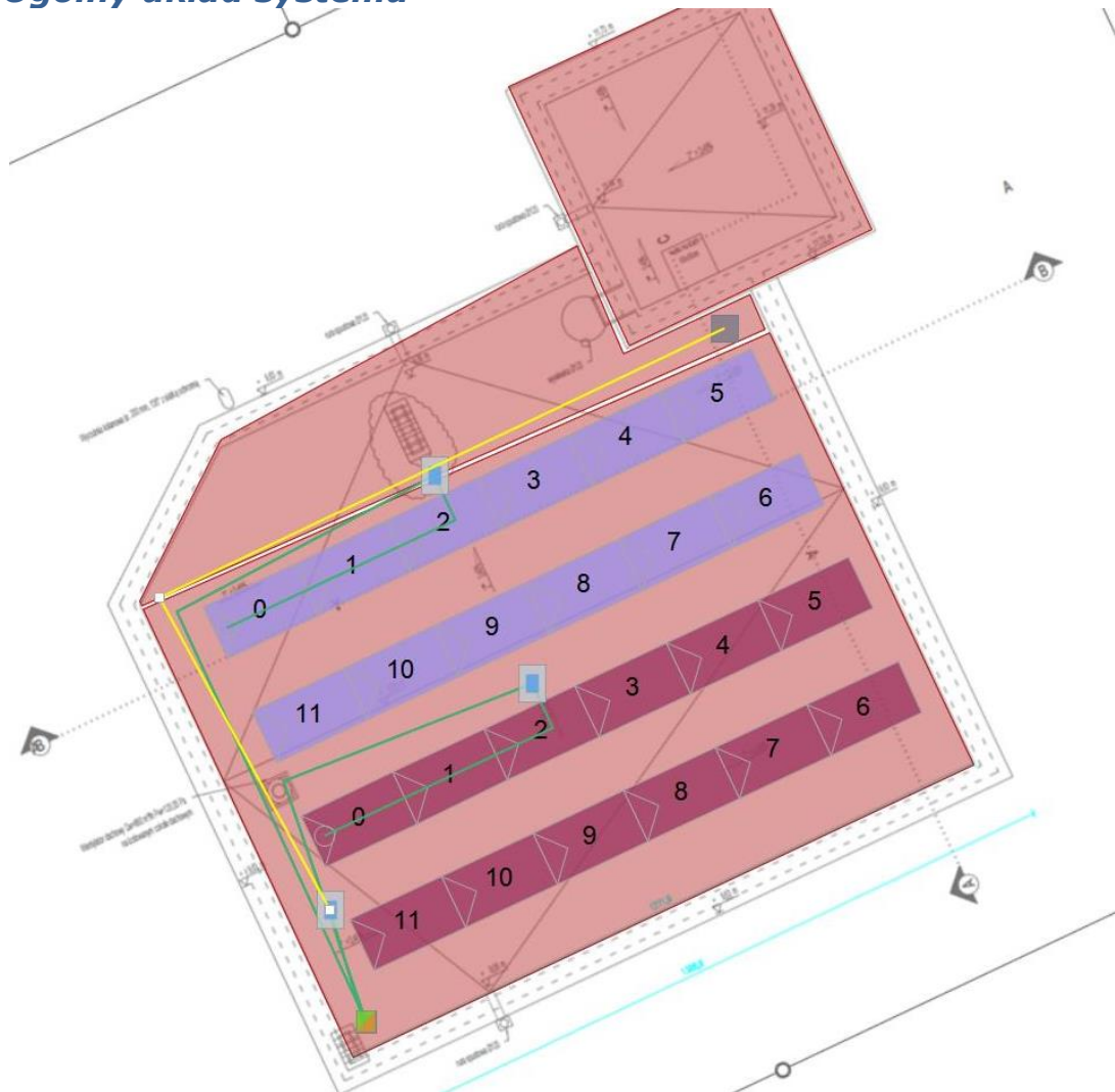
Rysunek 2: Umieszczenie generatora fotowoltaicznego i grupy przetwornic
