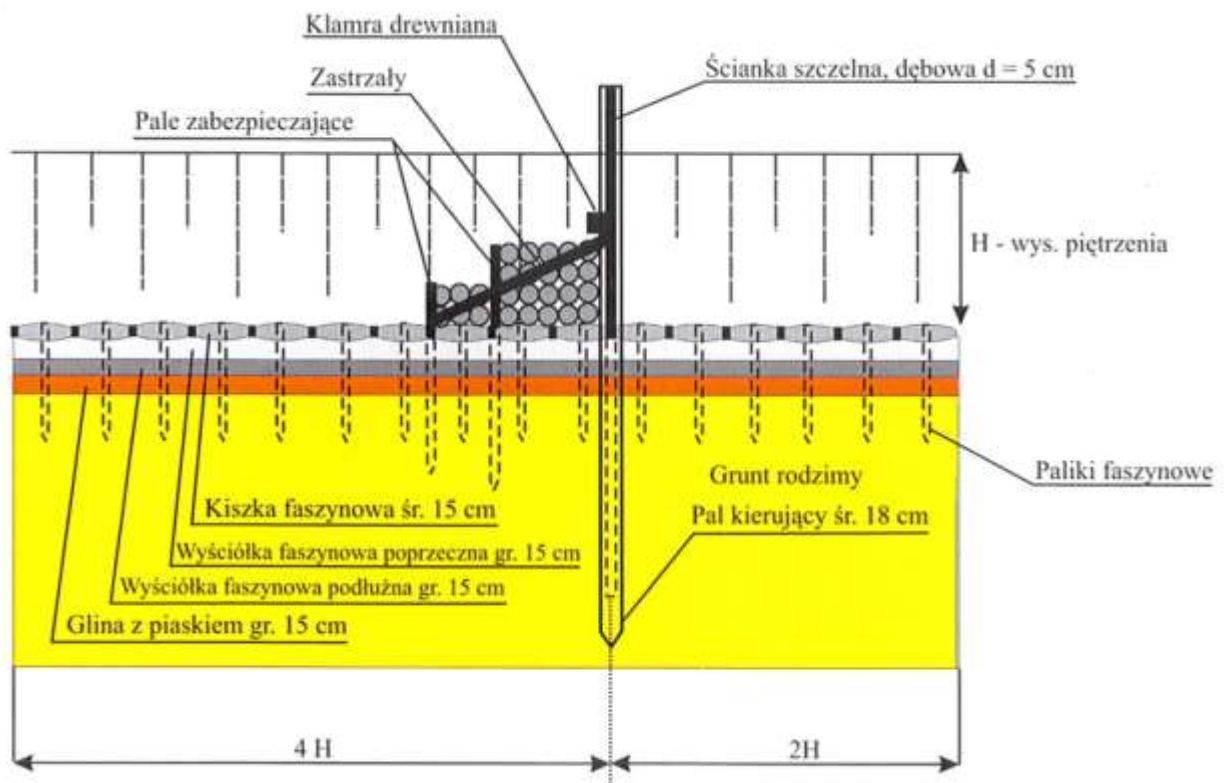
Przekrój podłużny przegrody o stałym poziomie piętrzenia umocnionej od strony wody dolnej. Źródło: M.Habichowa, P.Pawlaczyk, R.Stańko „Ochrona wysokich torowisk bałtyckich na Pomorzu”
