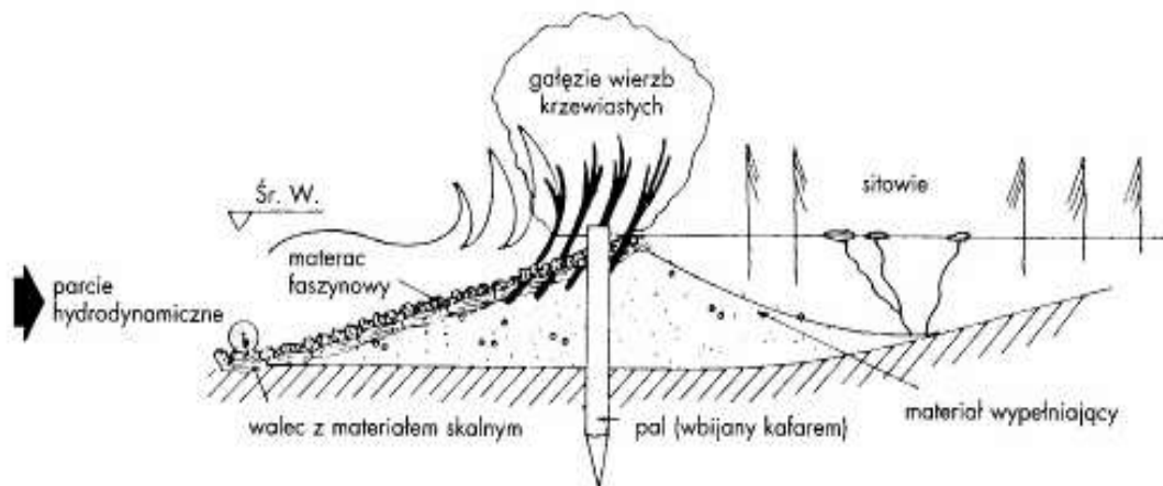
Tama faszynowa (Begemann i Schiechtel 1999)
