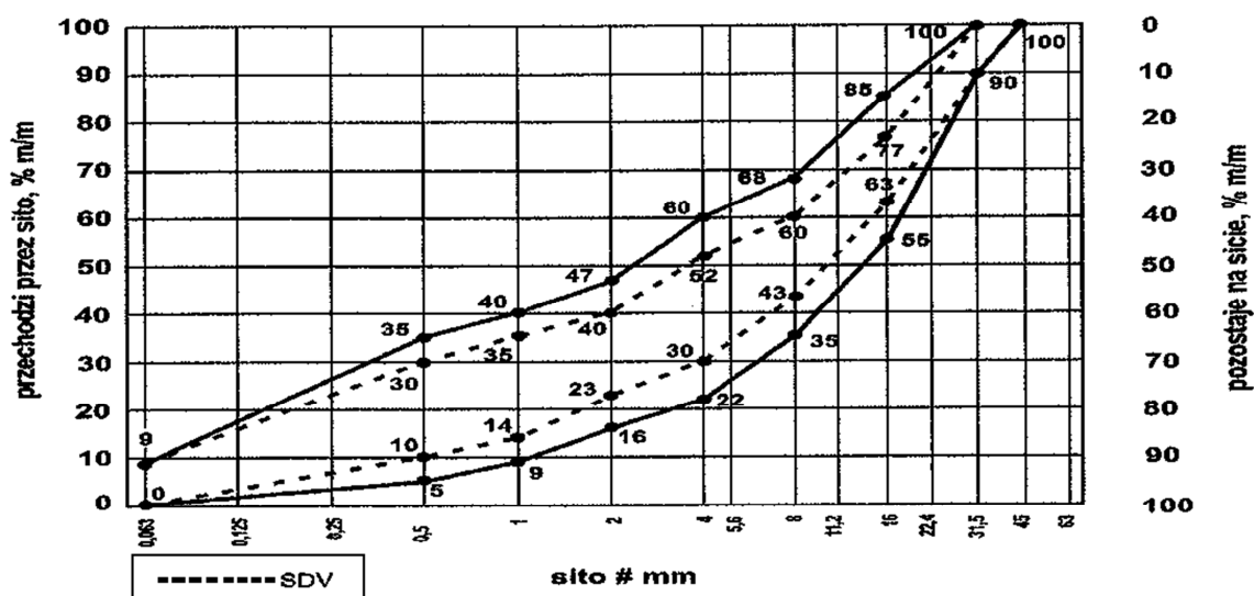
Rys. 1. Krzywe graniczne uziarnienia mieszanki kruszywo niezwiązanej 0/31,5 mm do warstw podbudowy zasadniczej
