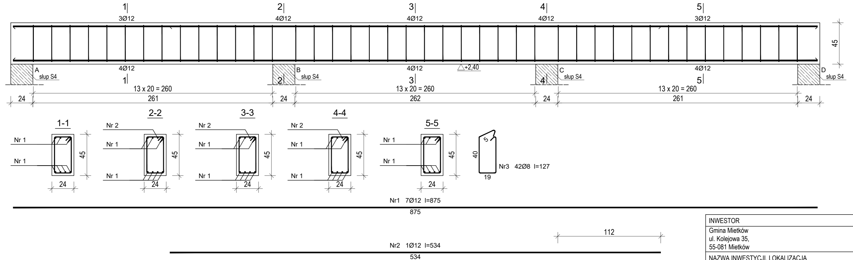
Wykaz zbrojenia
