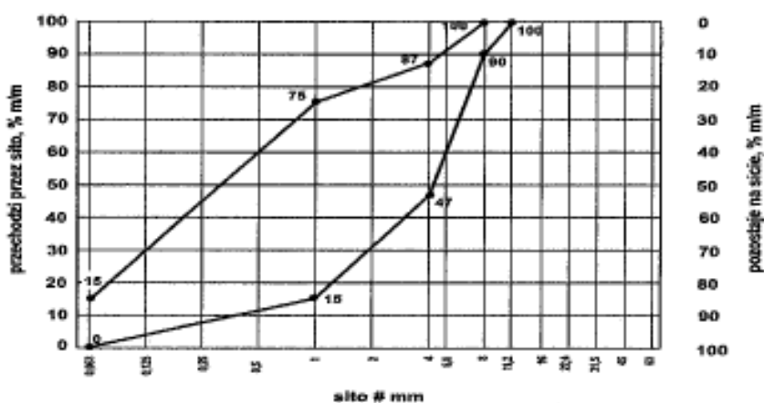
Rys. 2. Mieszanka kruszyw 0/8 do górnej warstwy podłoża ulepszonego
