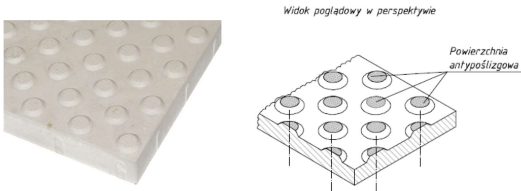
Rys. 2a. Płytki ostrzegawcze – szczegóły powierzchni
