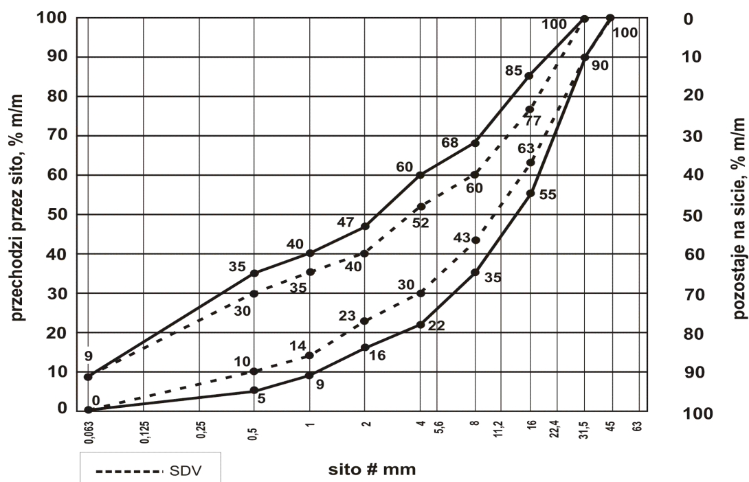
Rys. 5. Uziarnienie mieszanki niezwiązanej 0/31,5 dla podbudowy zasadniczej
