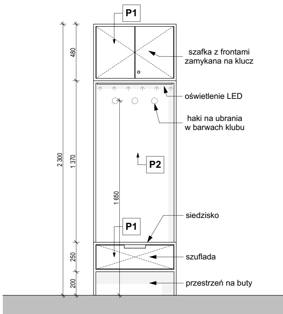
WIDOK 1:20
