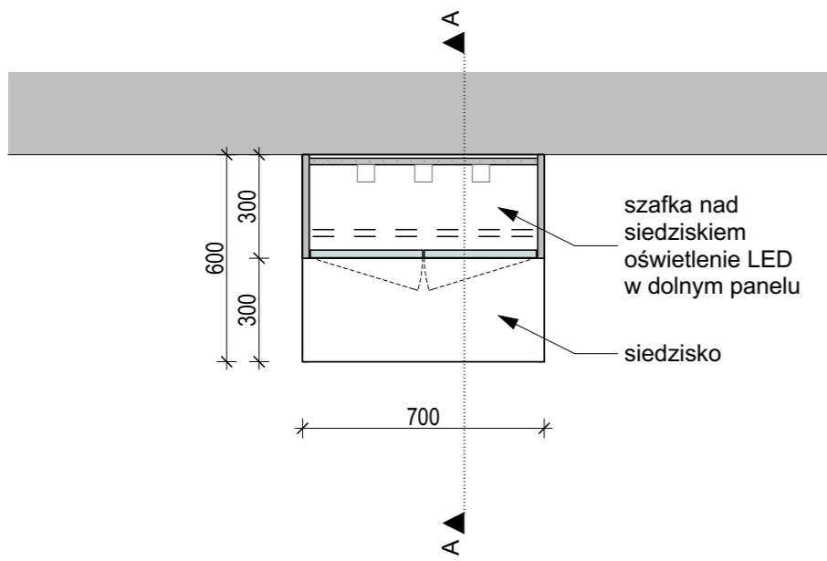
PLAN 1:20
